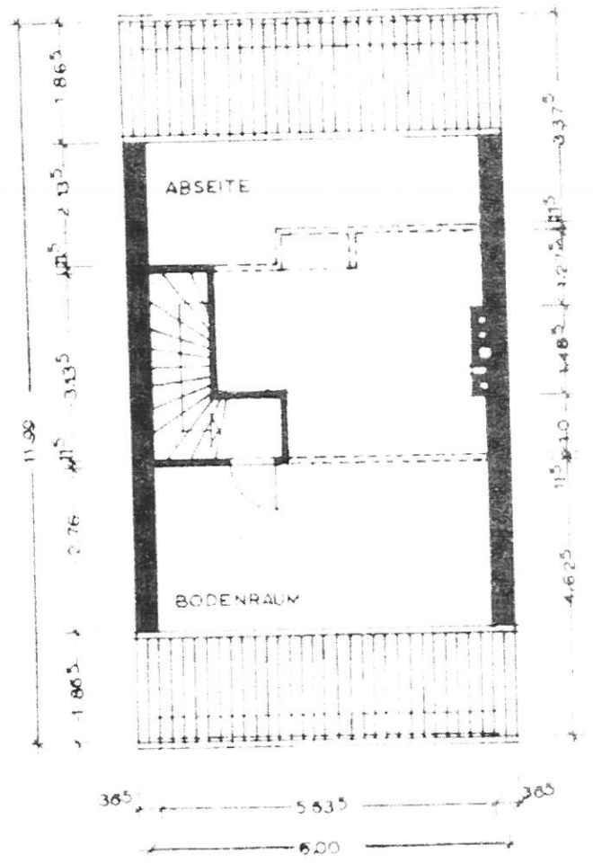
DACHGESCHOSS
