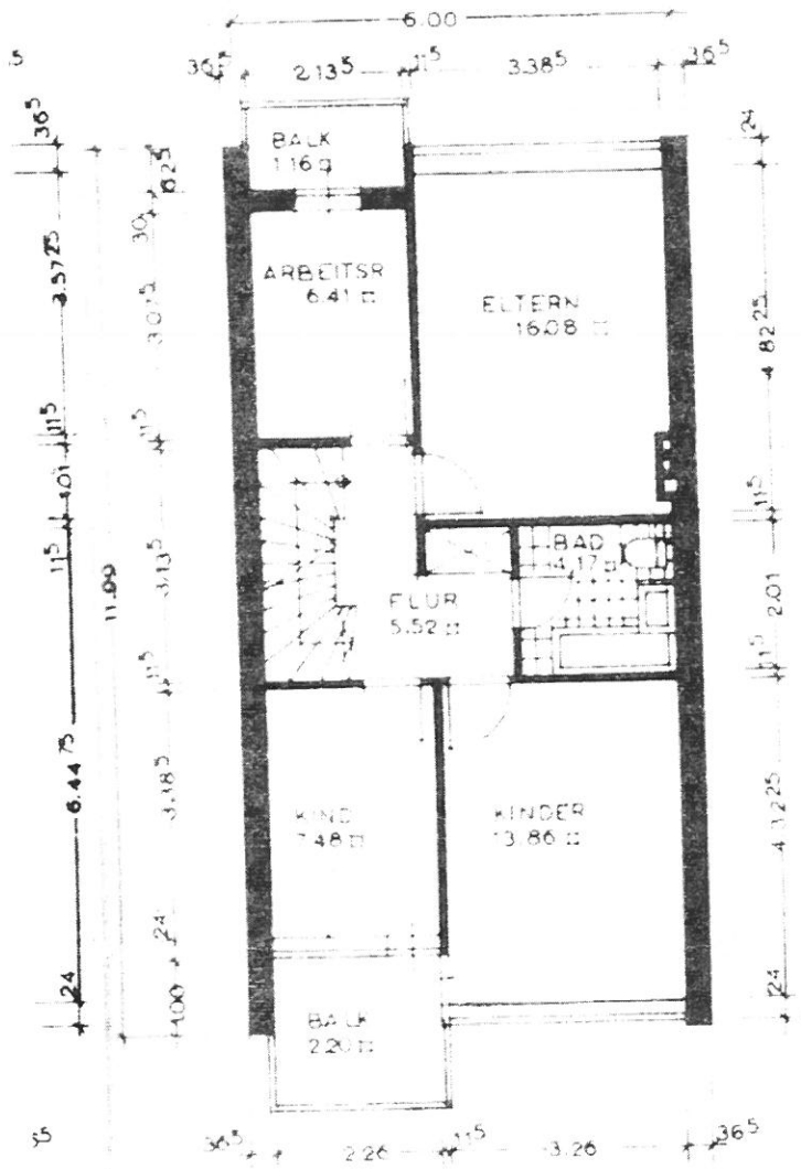
OBERGESCHOSS
